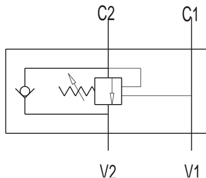
Hydraulisch Schema / Schéma hydraulique
