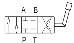
Hydraulisch schema Schéma hydraulique
